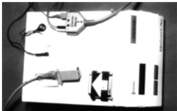
Fig. 1. Registradora portátil Eden Trace II Plus con los terminales del termistor, del pulsioxímetro y de los electrodos.
